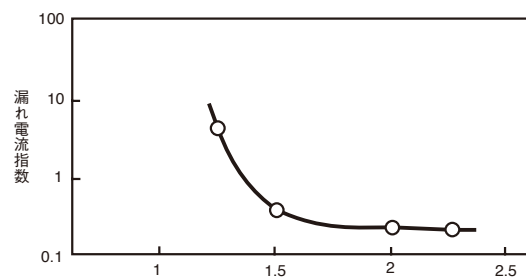
図3-5 電圧比
